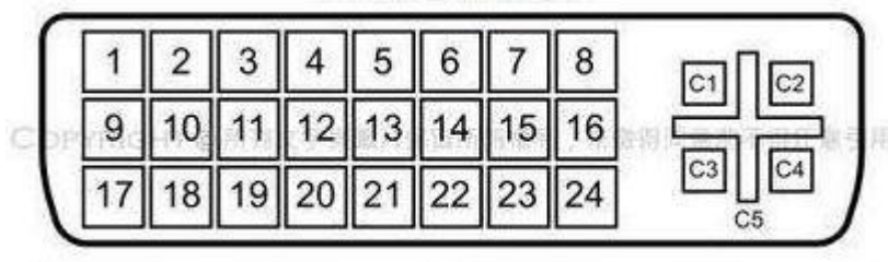
图 2.4.1 轴扩展接口引脚顺序
