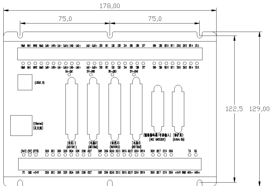
图 1.2.1 为 GCN400A(网络型控制器)的外观及尺寸:
