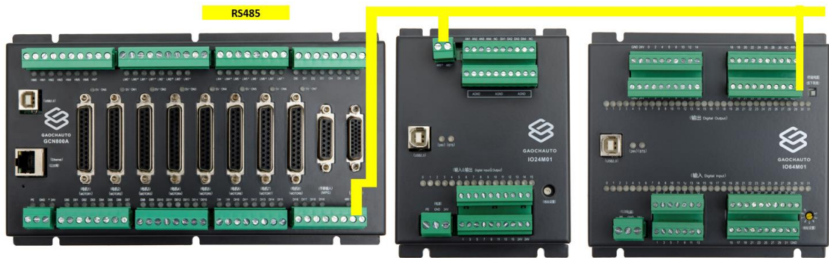
图 2.6.1 扩展模块接线示意图
