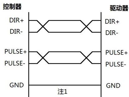
图 2.2.3 脉冲输出差分接法示意图
