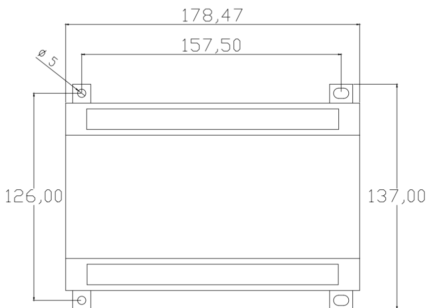
图 1.2.1 控制器尺寸图
