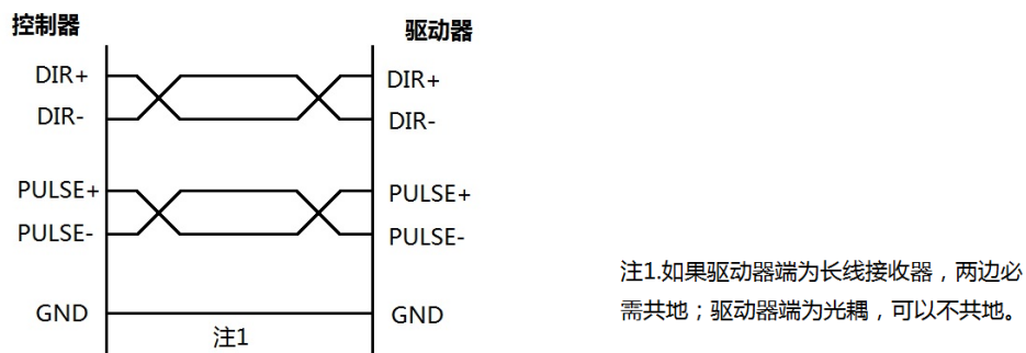
图 3.2.3 脉冲输出差分接法示意图
