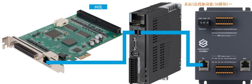
图 3.6.1 扩展模块接线示意图
