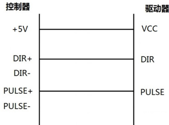
图 3.2.4 脉冲输出单端接法示意图
