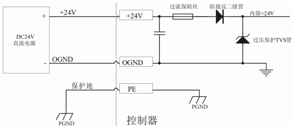
图 3.1.1 电源接口配线示意图
