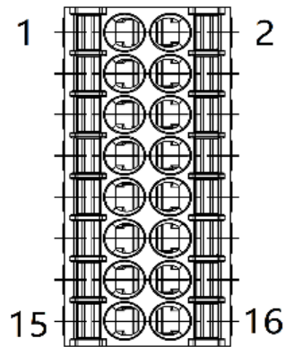
图 3.7.3 原点输入端子引脚顺序
