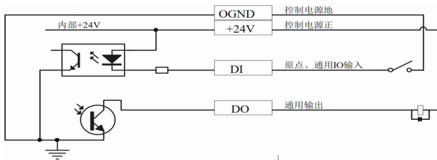
图 3.7.1 数字输入输出配线示意图
