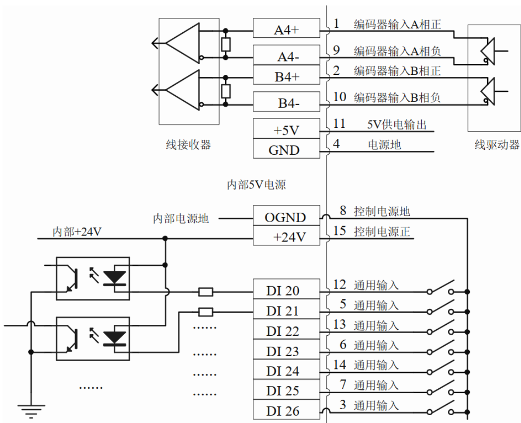
图 3.3.1 辅助编码器/手脉配线示意图
