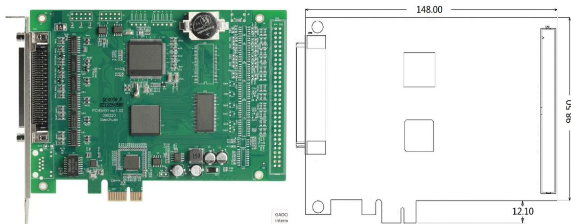
图 1.2.1 GCS400A-PCIE 控制卡主卡外观及尺寸图
