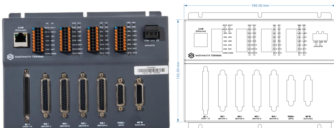
图 1.2.2 GCS400A-PCIE 控制卡端子板外观及尺寸图
