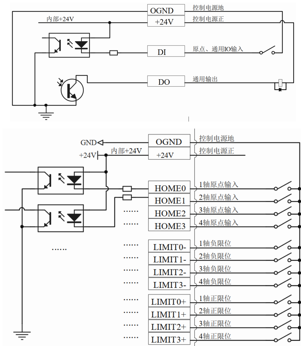
图 3.5.1 数字输入输出配线示意图
