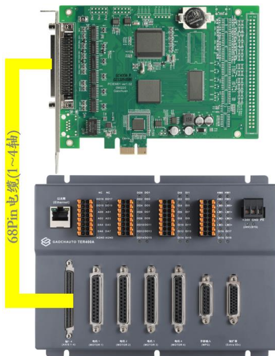
图 2.1.1 GCS400A-PCIE 控制卡与端子板连接示意图
