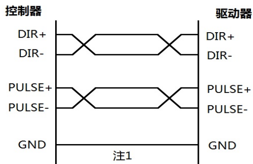
图 2.2.3 脉冲输出差分接法示意图
