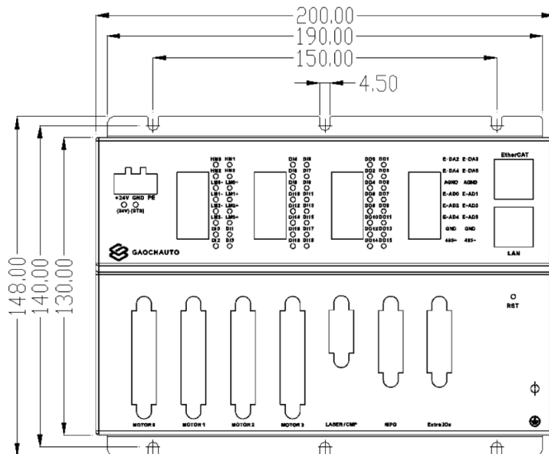
图 1.2.1 GCNH400A 的尺寸图
