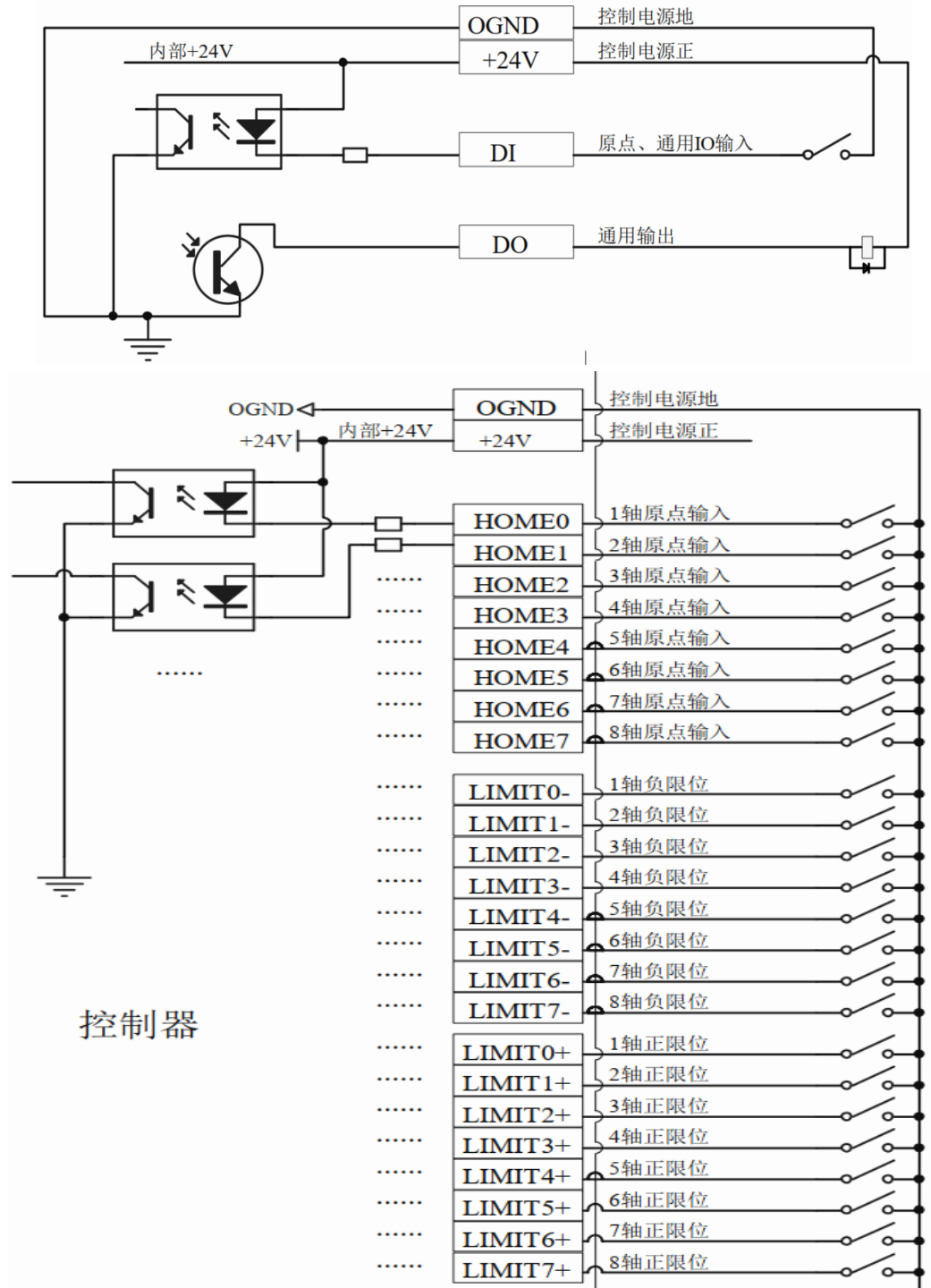
图 2.6.1 数字输入输出配线示意图
