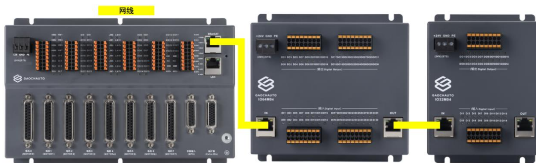
图 2.6.1 扩展模块接线示意图
