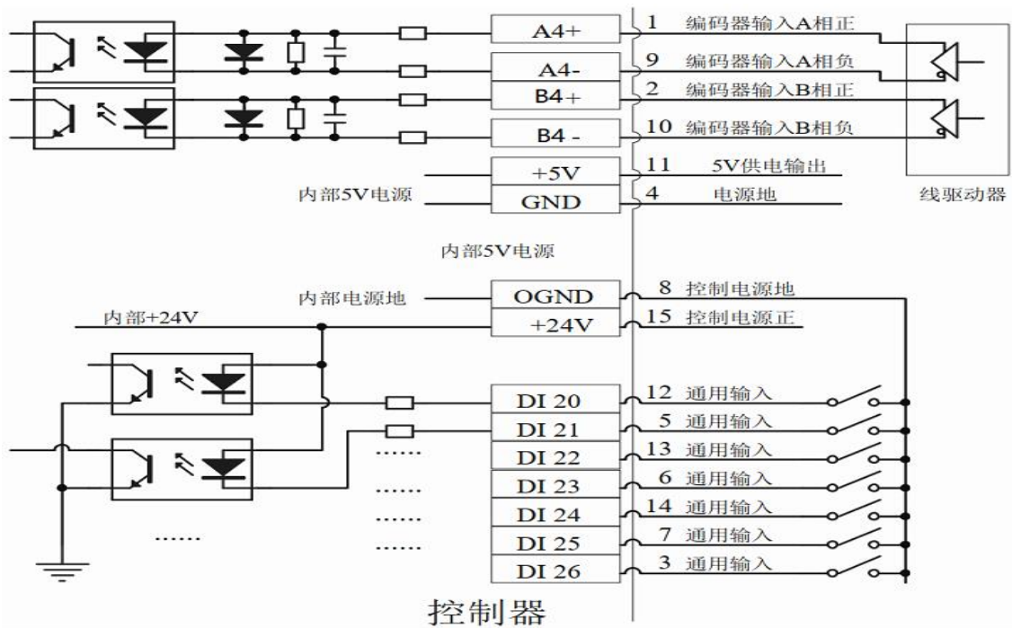
图 2.3.1 辅助编码器/手脉配线示意图
