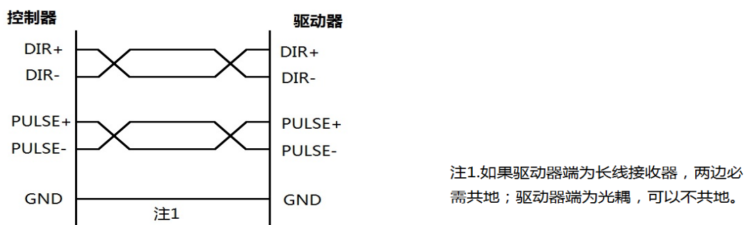
图 2.2.3 脉冲输出差分接法示意图
