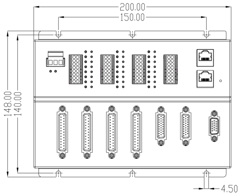
图 1.2.1 为 GCNH400A 的尺寸图，
