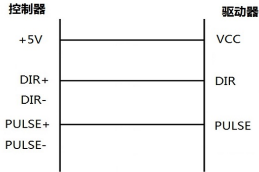
图 2.2.4 脉冲输出单端接法示意图
