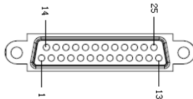
图 2.2.2 轴接口引脚顺序
