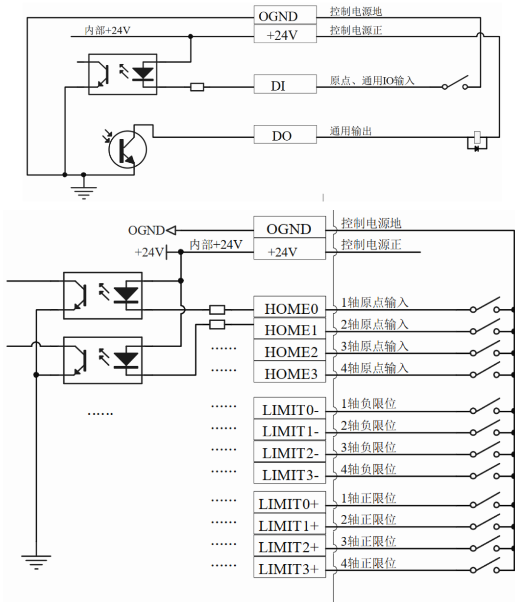
图 2.6.1 数字输入输出配线示意图
