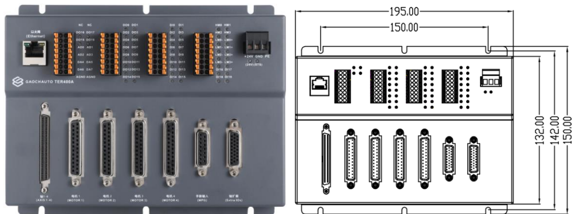
图 1.2.2 GCS400A-PCIE 控制卡端子板外观及尺寸图
