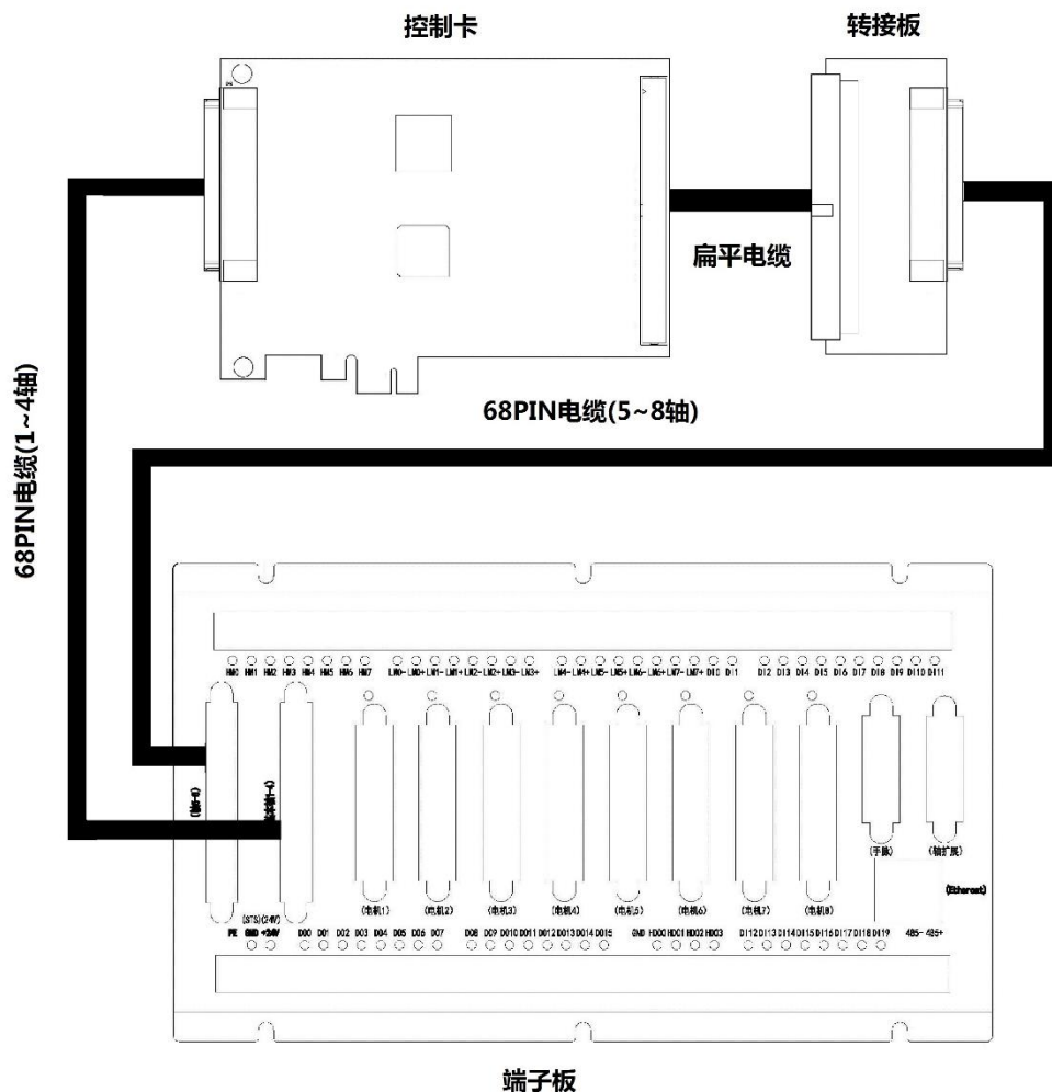
图 2.1.1 GC800A-PCIE 控制卡与端子板连接示意图
