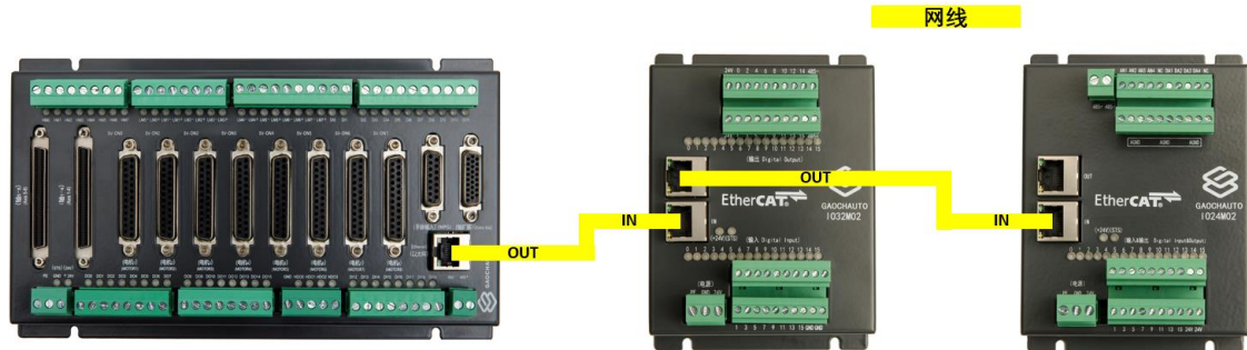
图 3.6.1 扩展模块接线示意图
