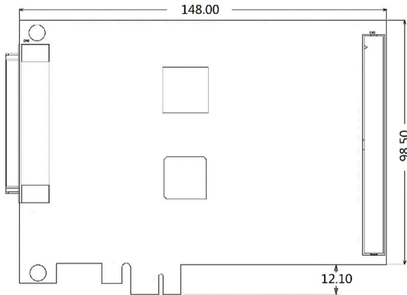
图 1.2.1 GC800A-PCIE 控制卡主卡外观及尺寸图
