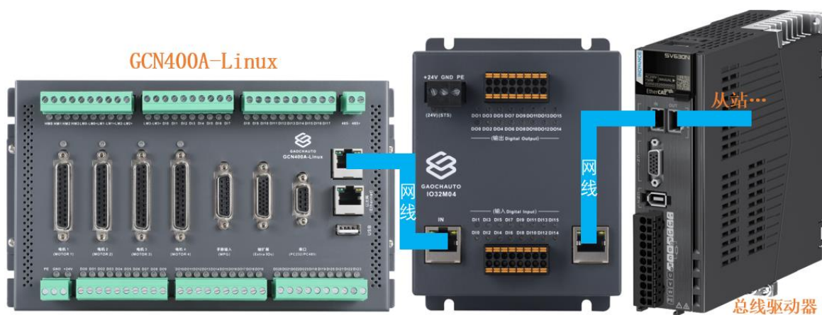
1.3.2 GCN400A-Linux 视觉控制器(特定型号) 设备控制接线图
