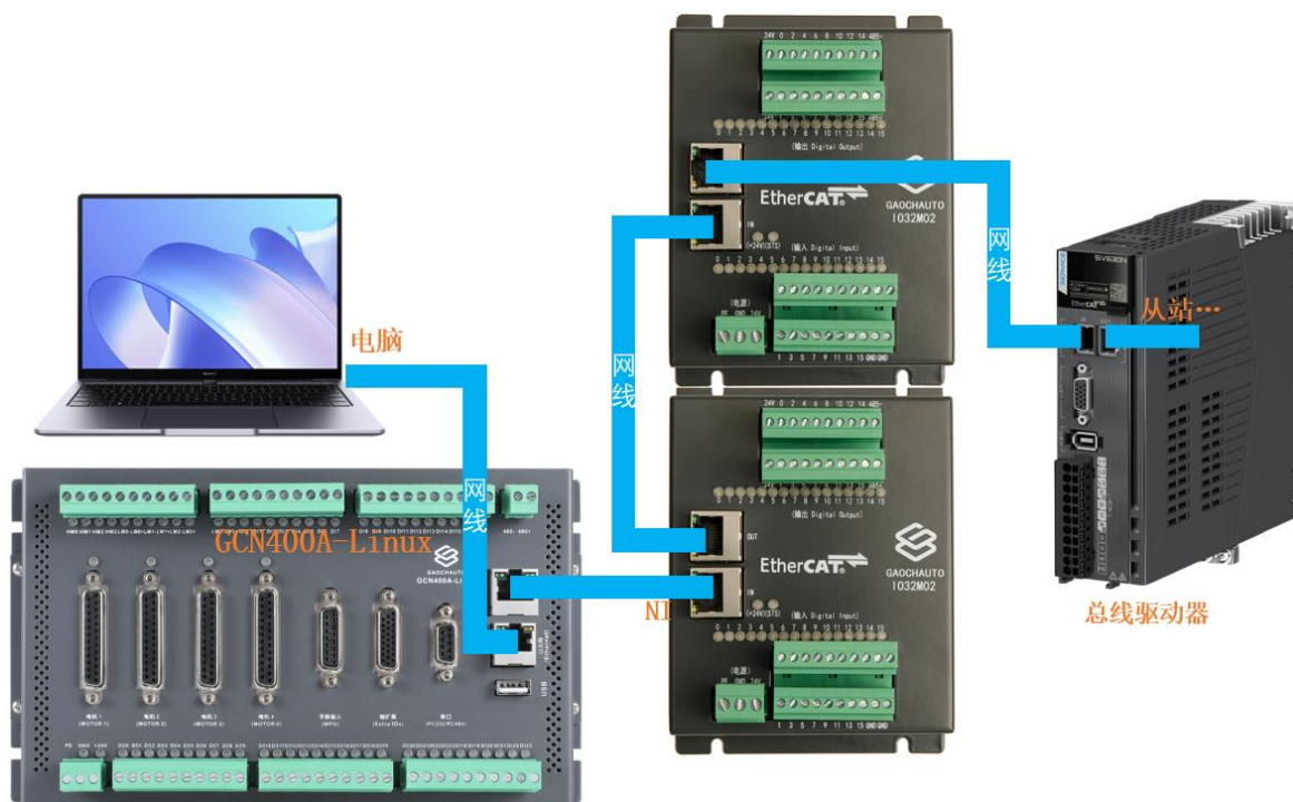
1.3.1 GCN400A-Linux 视觉控制器(特定型号)配置接线图
