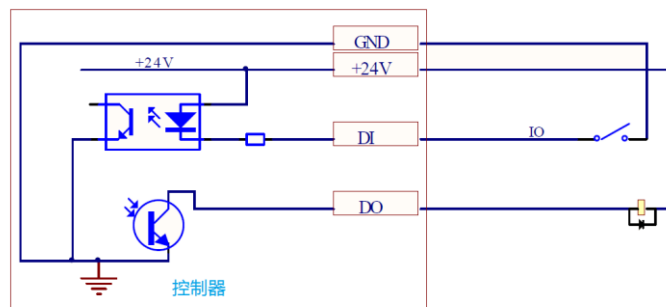
图 2.5.1 数字输入输出配线示意图
