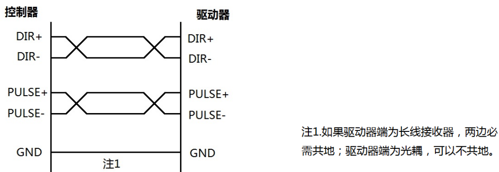
图 2.2.3 脉冲输出差分接法示意图
