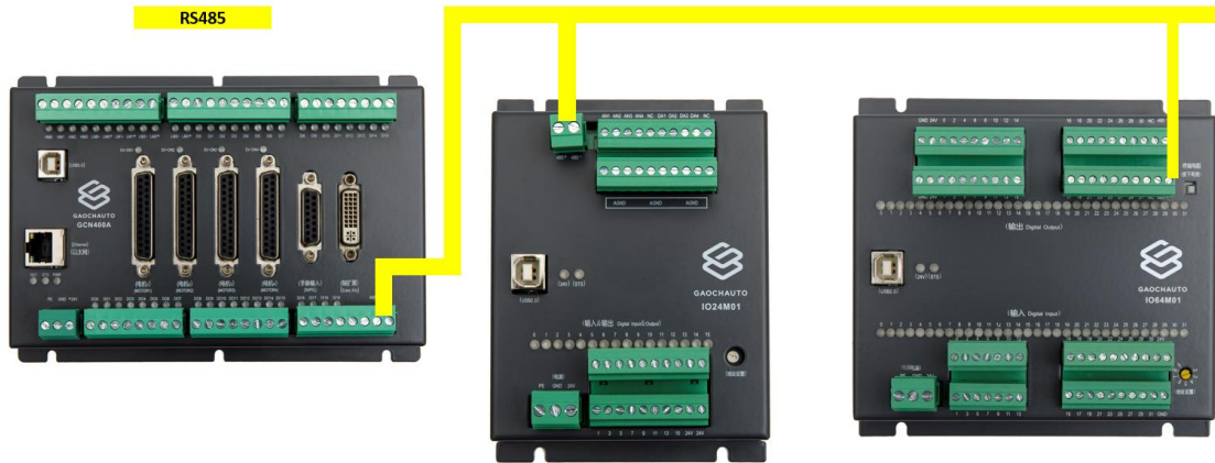
图 2.6.1 扩展模块接线示意图
