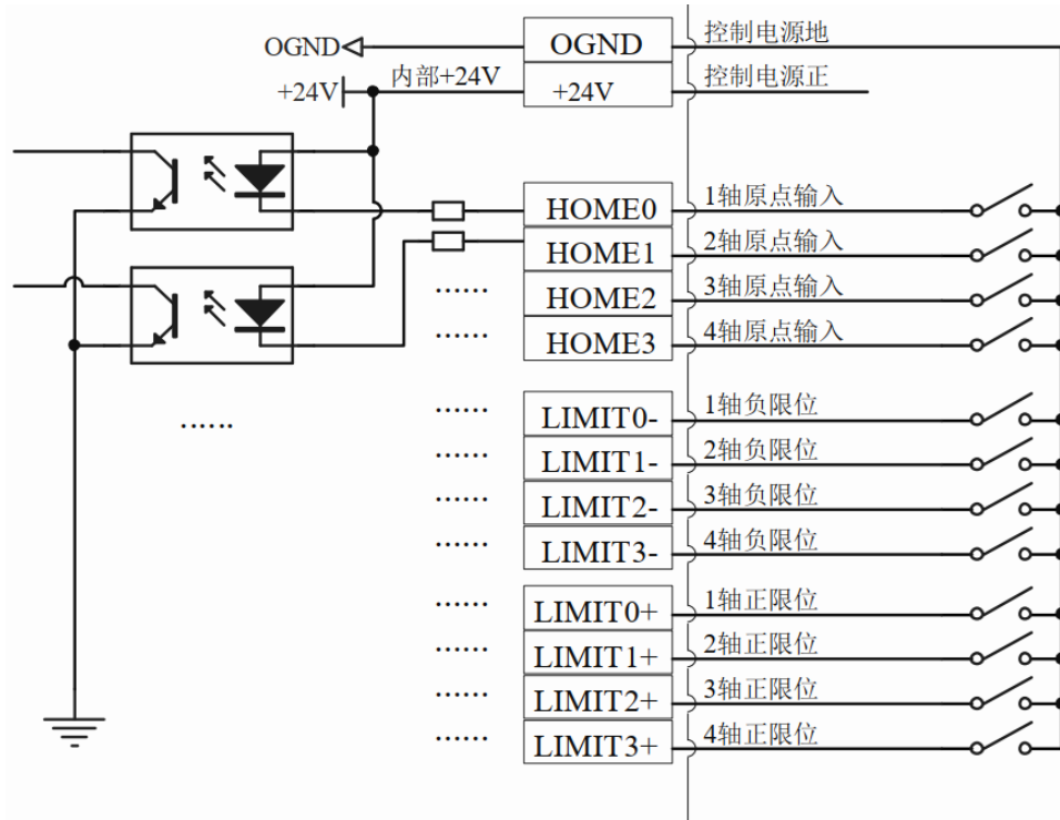
图 2.5.1 数字输入输出配线示意图
