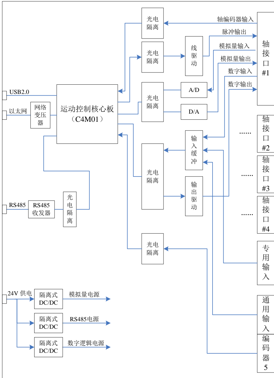
图 1.2.1 控制器的系统框图
