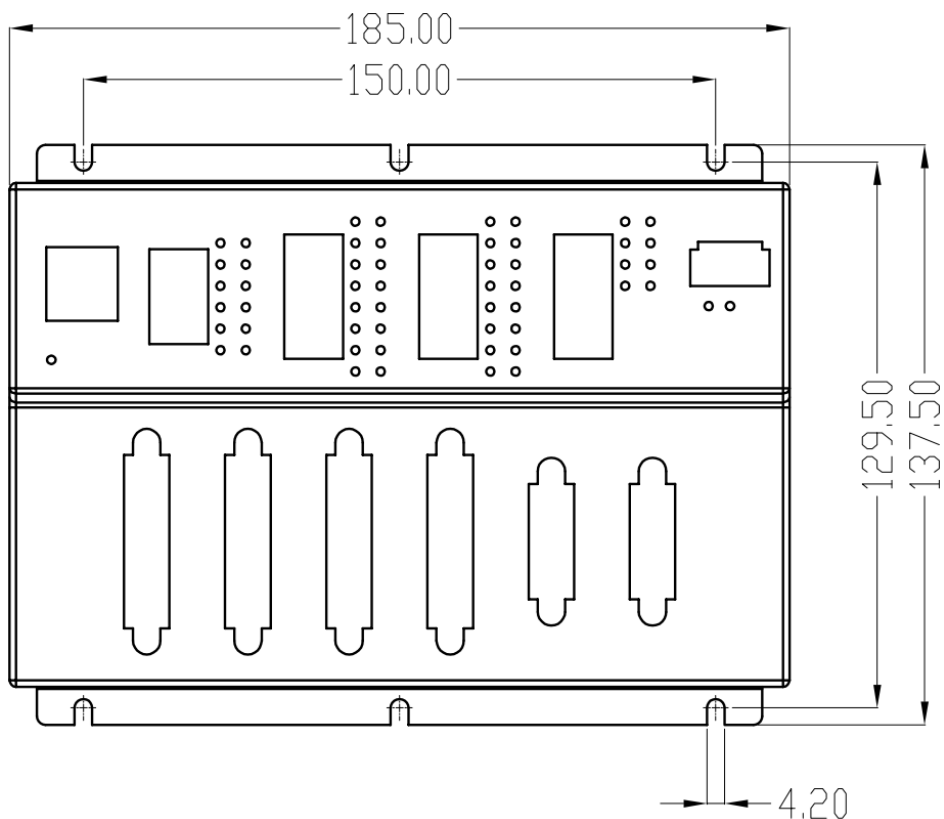
图 1.1.1 控制器尺寸图
